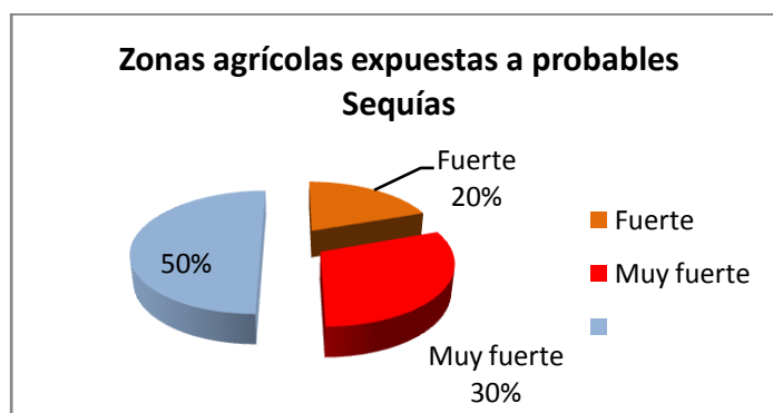
Figura 35.- Porcentajes de áreas agrícolas expuestas a las zonas de mayor probabilidad de sequías en el municipio de Zacatlán
